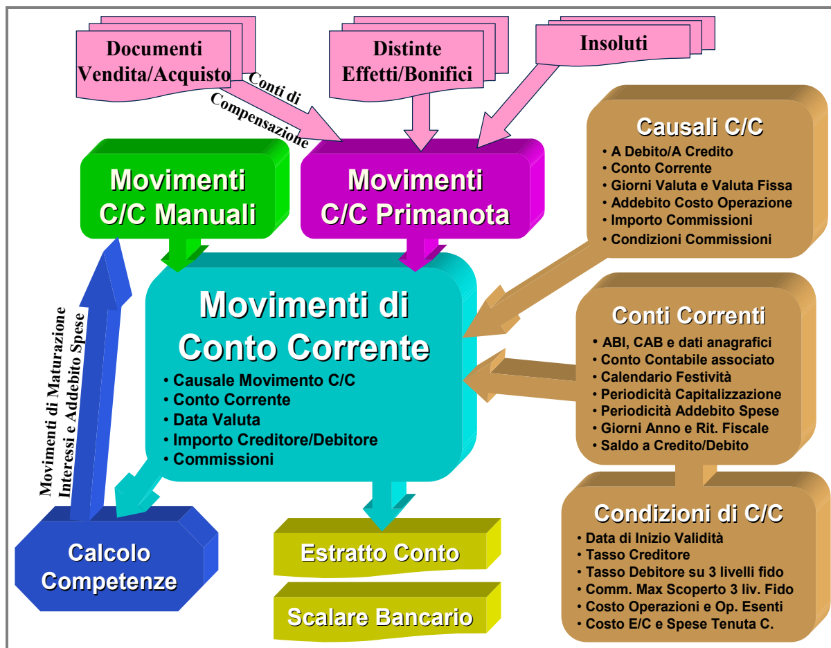
Fig. 1.1 – Schema logico del modulo Conti Correnti
