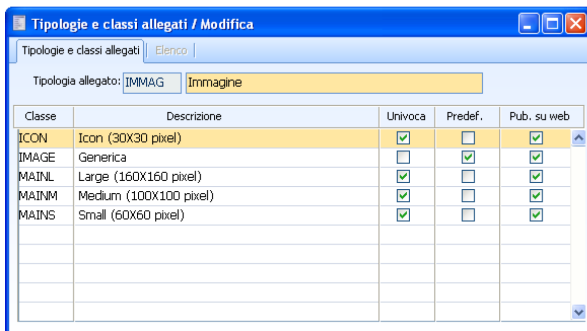
Fig. 3.22 – Tipologie Allegati
