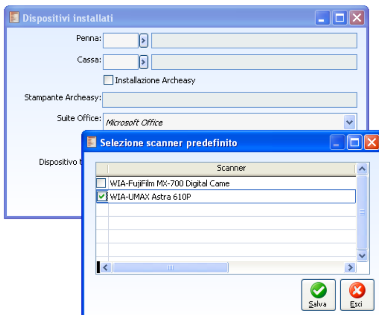
Fig. 3.7 - Selezione Scanner.
