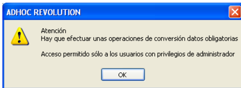
Fig. 5.6 – Messaggi tradotti.
