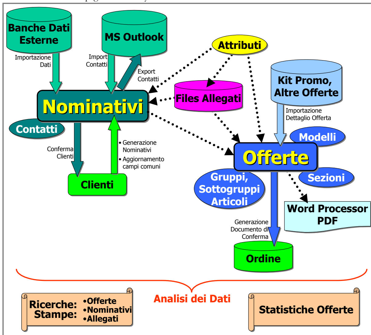
Fig. 1-1 – Struttura funzionale del modulo Offerte
