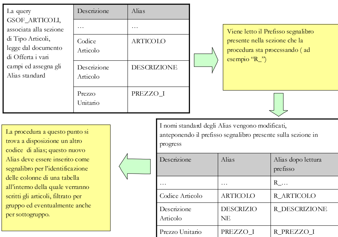
Fig. 2-17 - Metodo di applicazione dei Prefissi Segnalibro.
