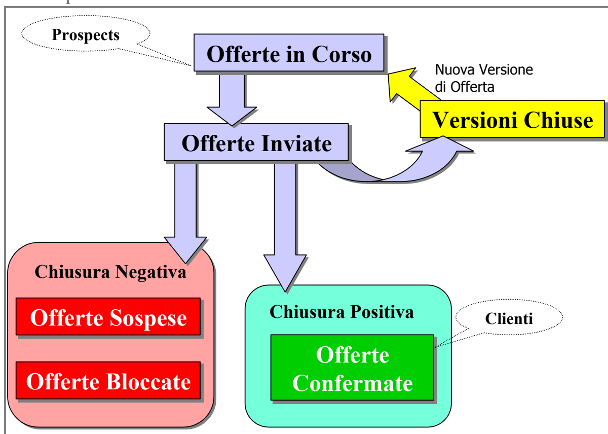
Fig. 1-3 – Pipeline dell'Offerta
