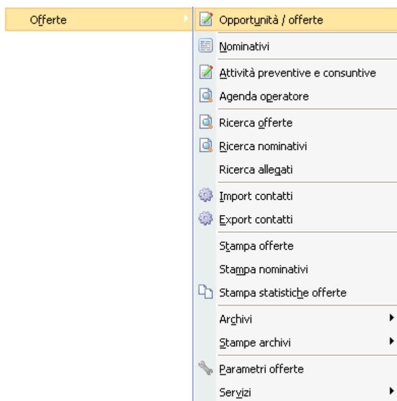
Fig. 2-1 - Menu Archivi
