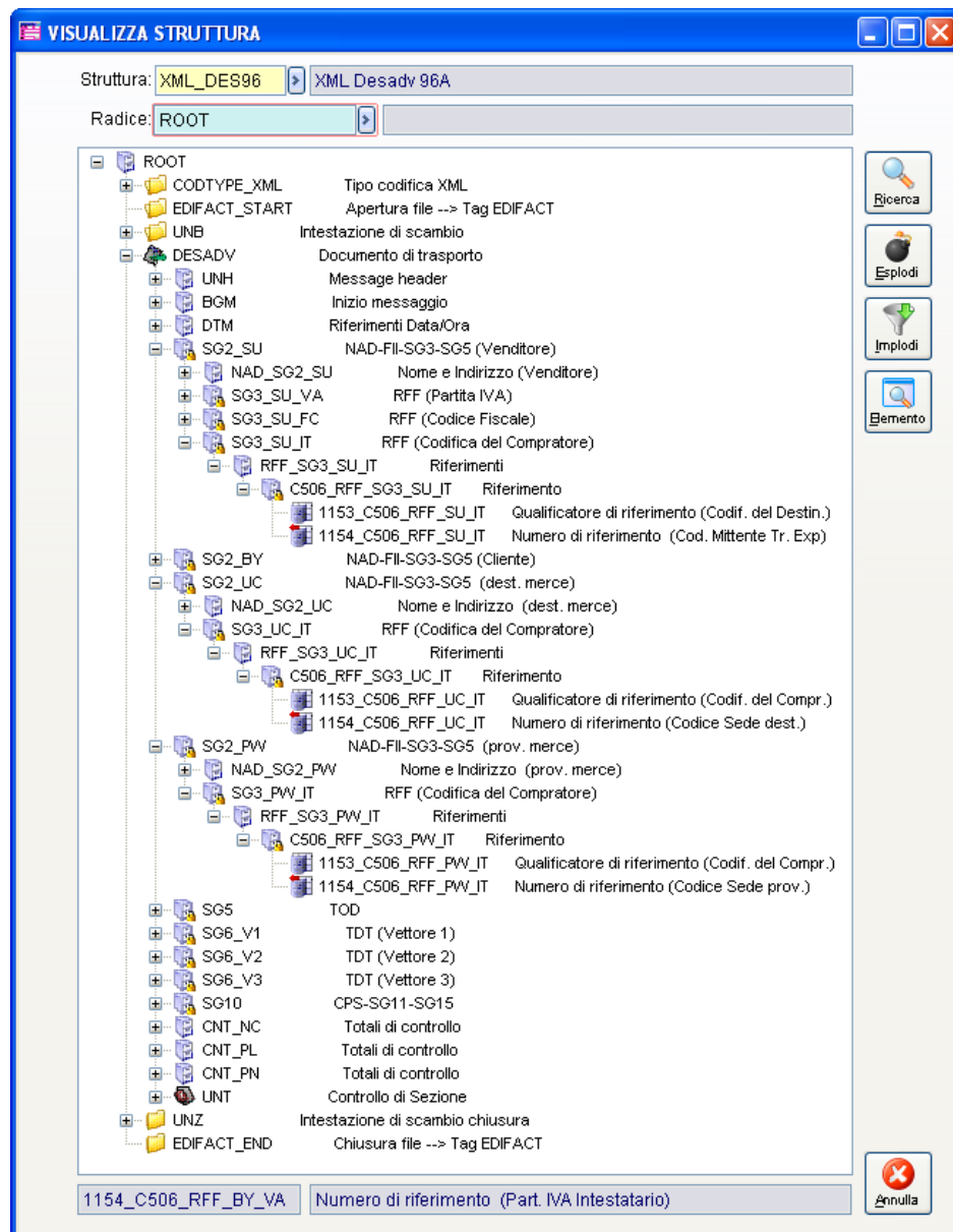
Fig. 2.50 – Treeview con esplosione del gruppo SG2_SU
