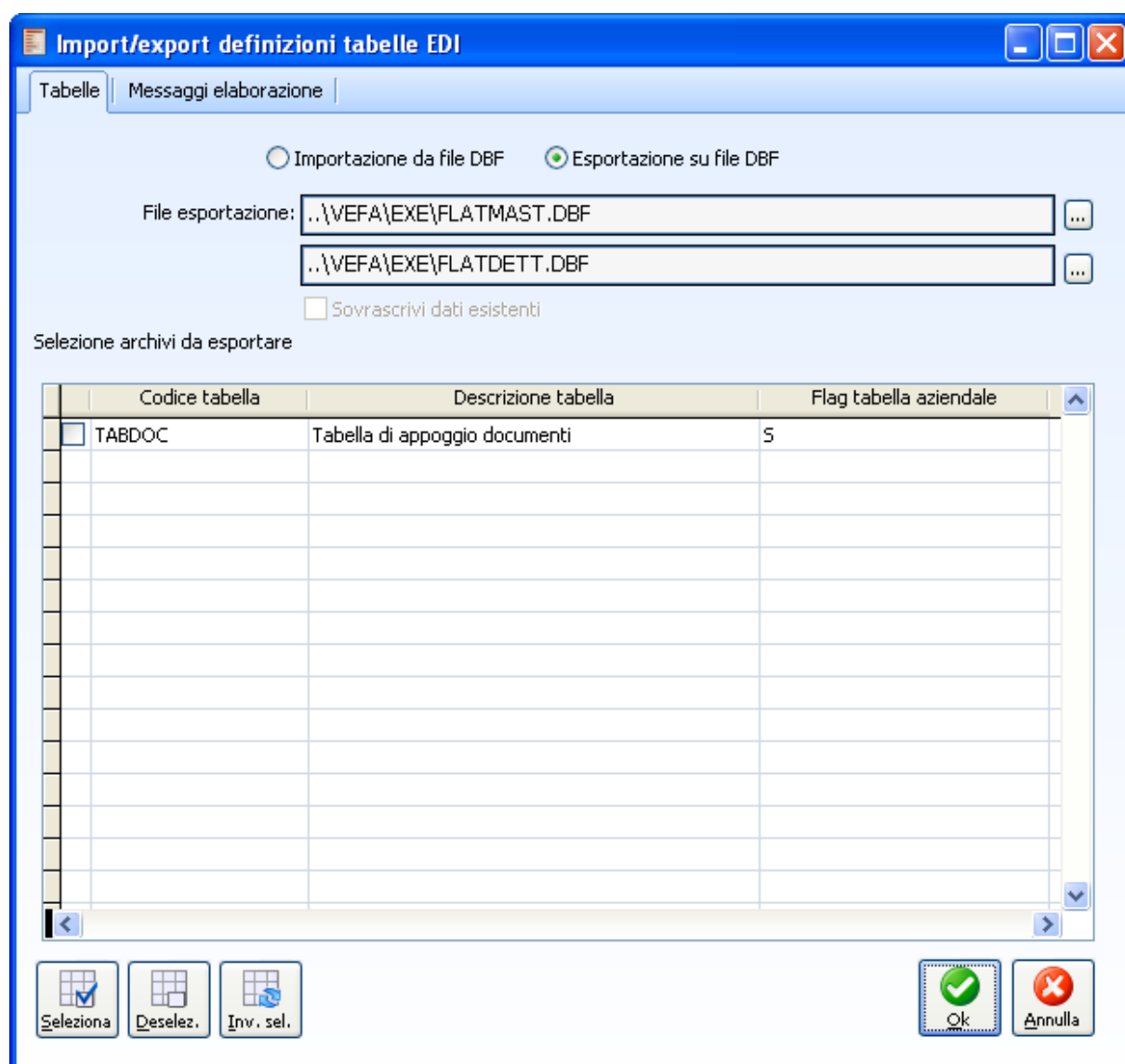
Fig. 2.64 – Import/Export tabella piatta
