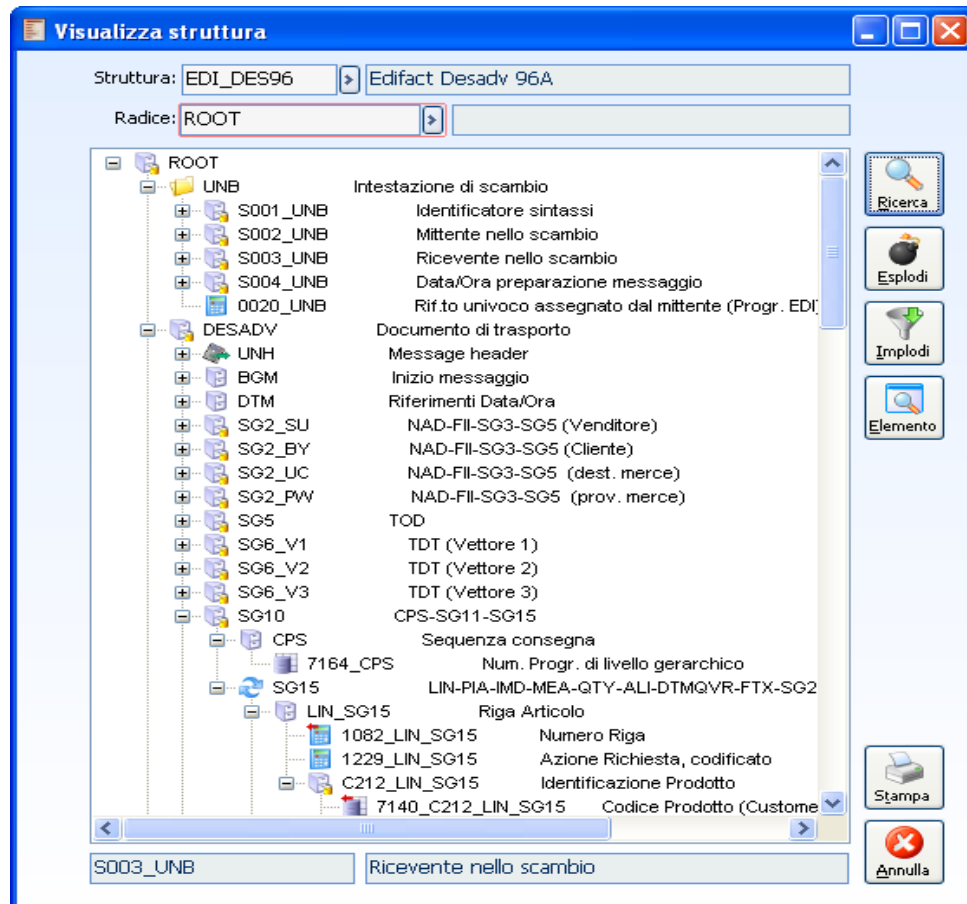
Fig. 2.38 – Treeview struttura EDI
