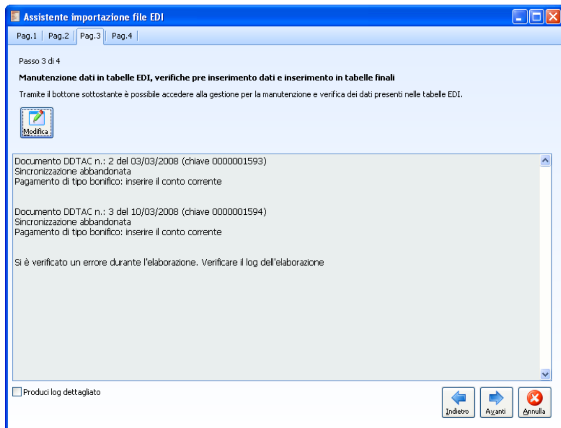
Fig. 2.53 - Assistente Importazione Files EDI –Step 3
