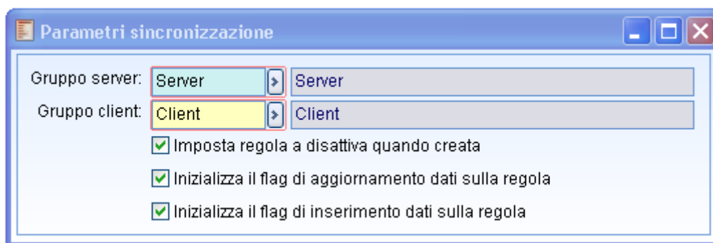
Fig. 1-9 – Parametri sincronizzazione
