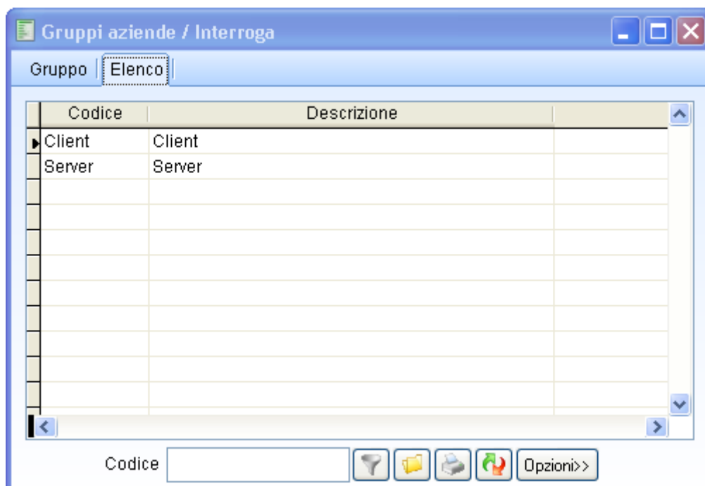
Fig. 1-6 – Gruppi “elenco”
