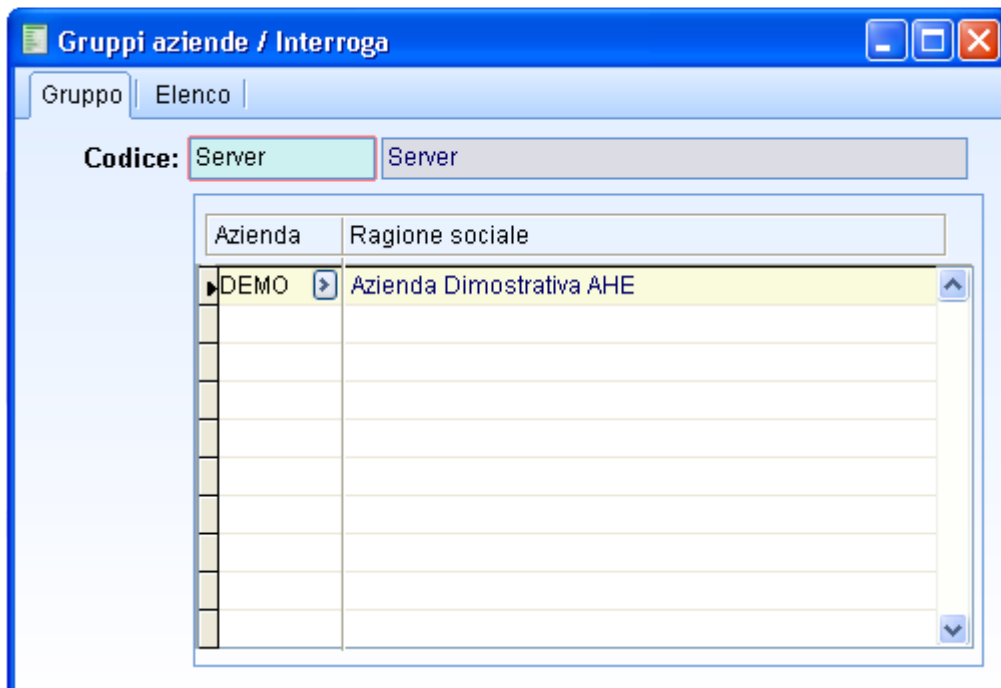
Fig. 1-7 – Gruppi “server”
