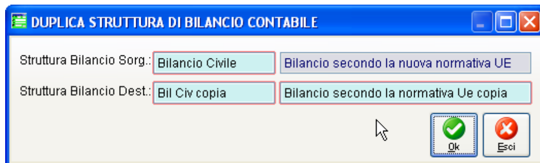
Fig. 4.44 – Duplica Struttura
