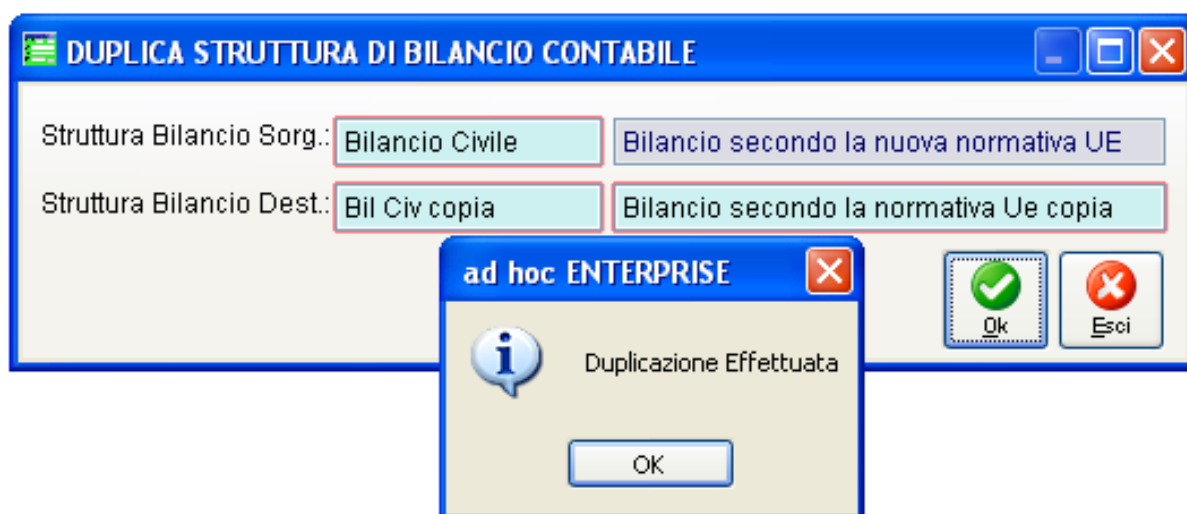
Fig. 4.45 – Duplica Struttura
