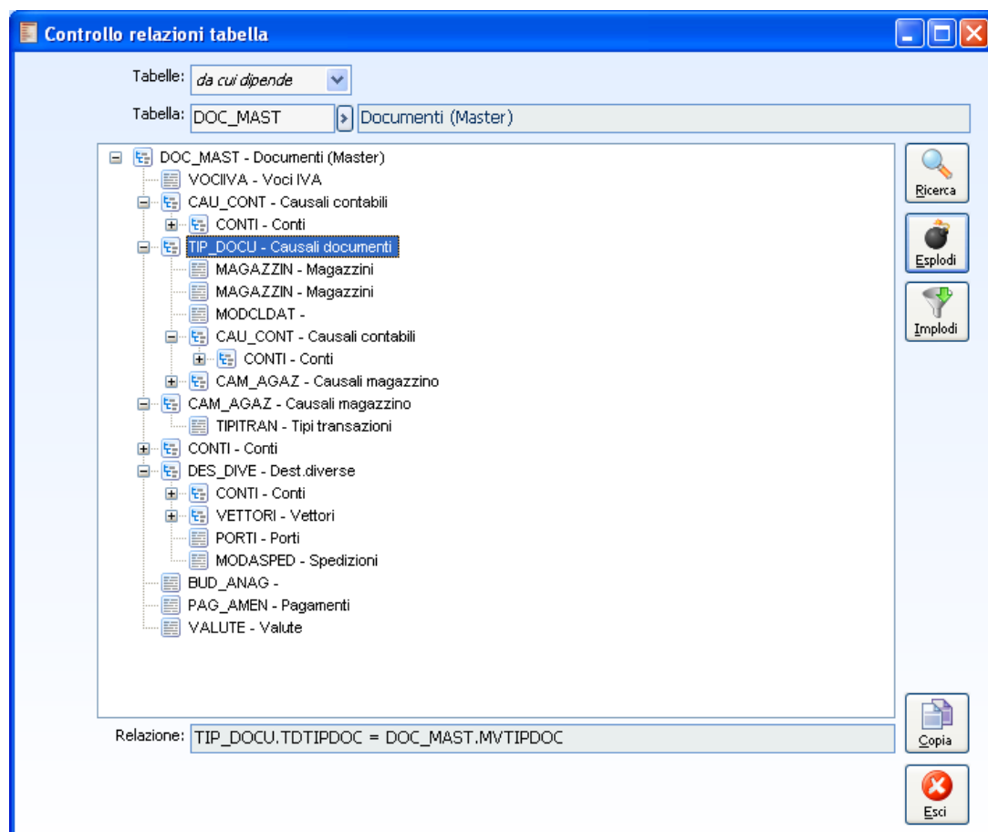
Fig. 1-8 – Controllo Relazioni Tabella
