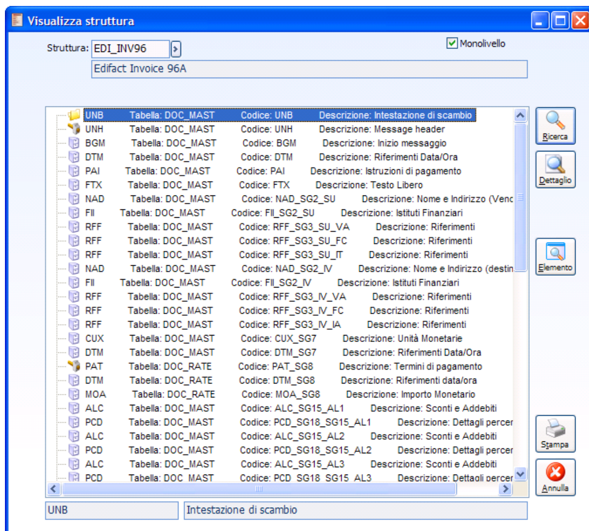
Fig. 1-39 – Treeview struttura EDI
