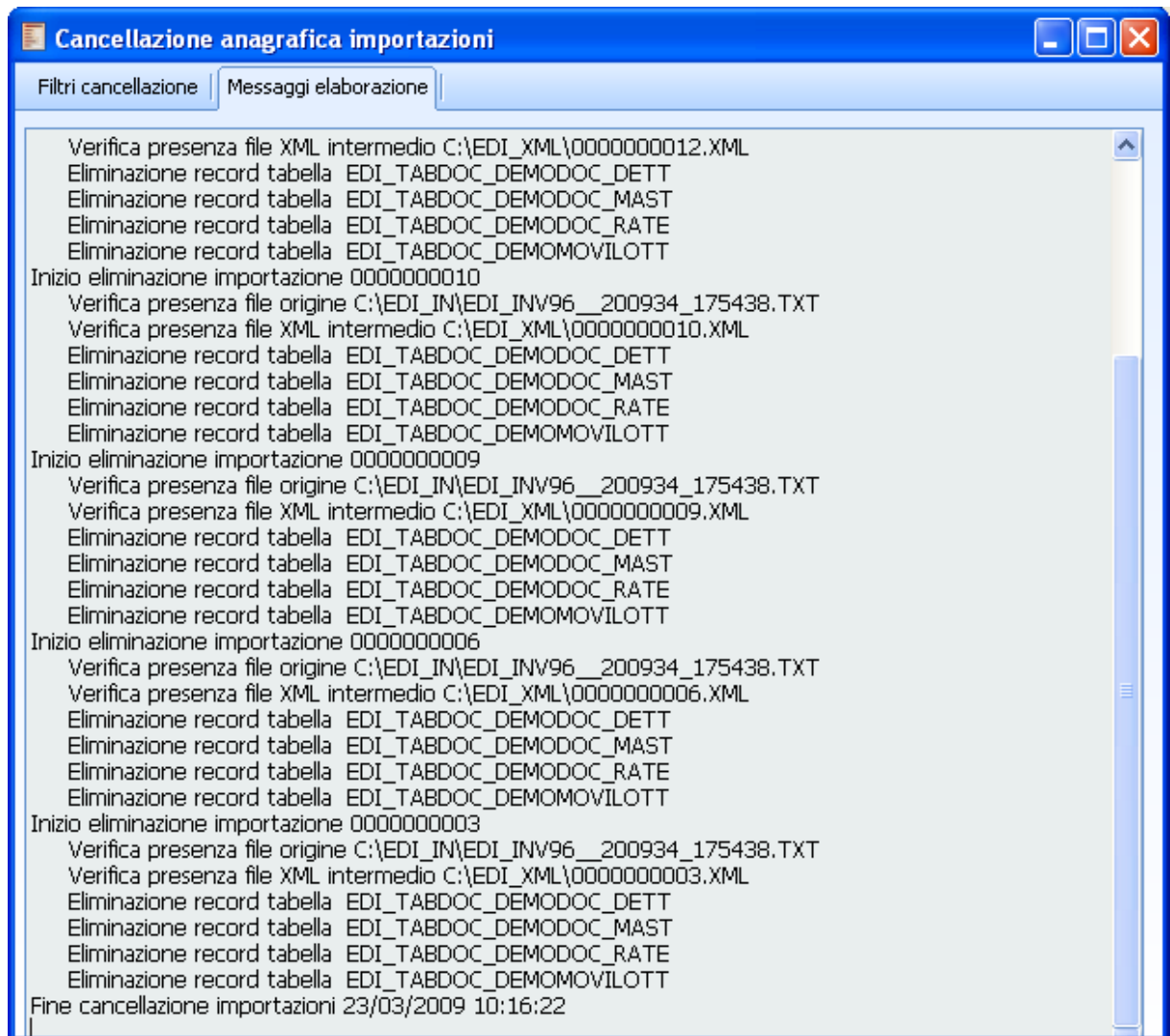
Fig. 2-22 – Messaggi elaborazione
