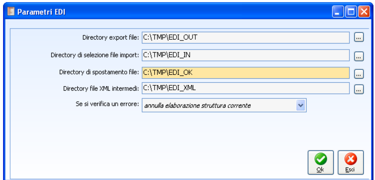
Fig. 1-16 – Parametri EDI
