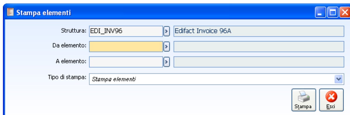
Fig. 1-24 – Stampa Elementi
