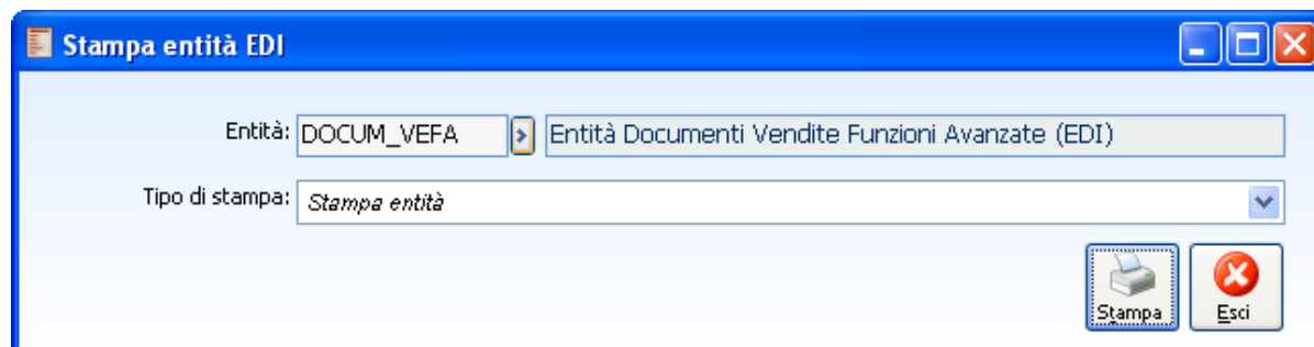
Fig. 1-23 – Stampa Entità
