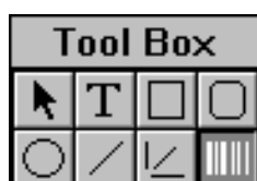
Fig. 8.16 - Toolbox
