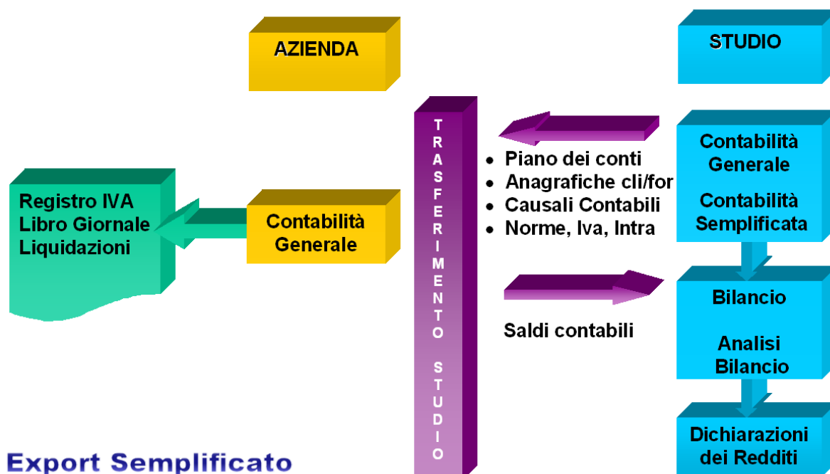
Flusso Schematico Dati Modalità Semplice
